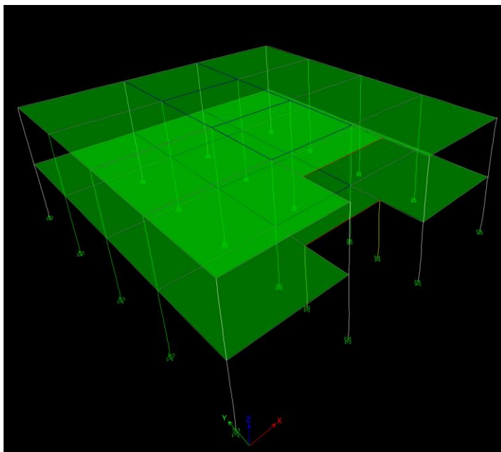
-Modul 1 de vibrație-Translatie Y;T=0.422-
