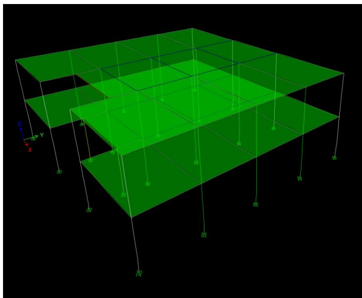
Modul 2 de vibrație-Translatie X ;T=0.406-
