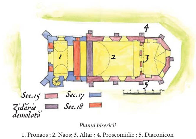
Planul bisericii 1. Pronaos ; 2. Naos; 3. Altar ; 4. Proscomidie ; 5. Diaconicon
